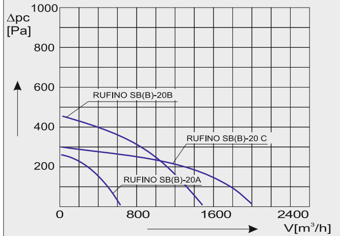
Charakterystyka aerodynamiczna RUFINO SB(B)-20
