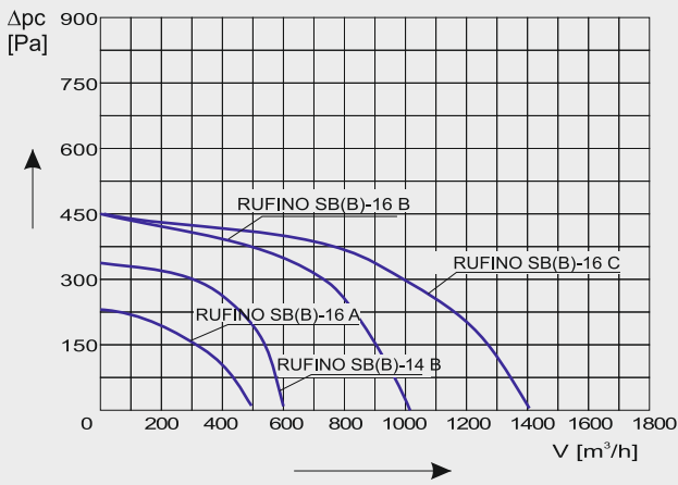
Charakterystyka aerodynamiczna RUFINO SB(B)-14,16
