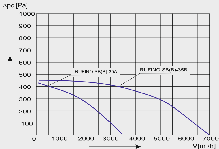
Charakterystyka aerodynamiczna RUFINO SB(B)-35
