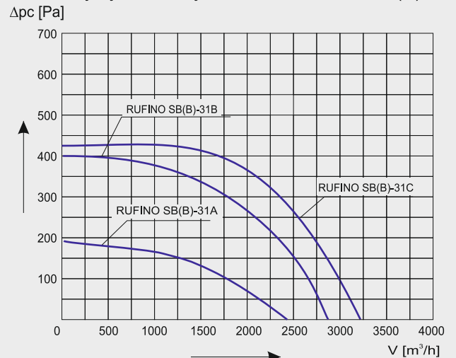
Charakterystyka aerodynamiczna RUFINO SB(B)-31
